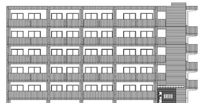
南西側立面図 S=1:150
